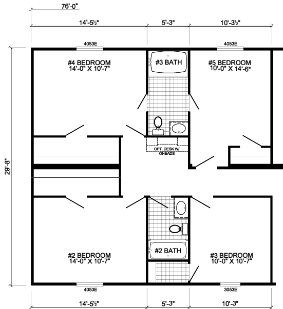
OPTIONAL 4'-0" STRETCH
